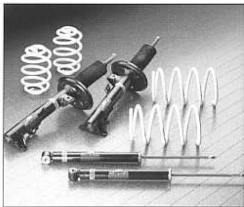
AC Schnitzer Sportfahrwerk (Abstimmung sportlich komfortabel) oder AC Schnitzer Fahrwerks-Federsatz für Fahrzeuge mit oder ohne M-Technik Stoßdämpfer.
